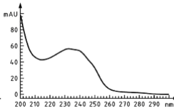
b) Espectro de absorción típico de MC-YR en un sistema d acetonitrilo/agua
